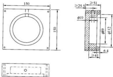
图 7.2.2-2 试验槽示意图(mm)
