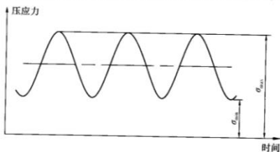
图 13.0.4 试验荷载示意图
