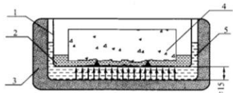
图 4.3.3-5 试件盒在超声浴槽中的位置示意图(mm) 1—试件盒; 2—试验液体; 3—超声浴槽; 4—试件; 5—水
