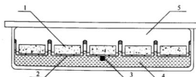
图 4.3.3-3 单面冻融试验箱示意图 1—试件；2—试件盒；3—测温点(参考点)； 4—制冷液体；5—空气隔热层
