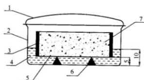
图 4.3.3-1 试件盒示意图(mm) 1—盖子；2—盒体；3—侧向密封；4—试验液体； 5—试液表面；6—垫条；7—试件
