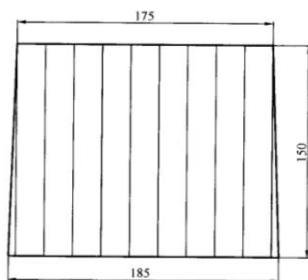
图 6.1.2 梯形板示意图(mm)
