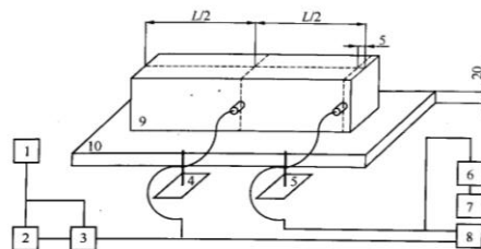
图 5.0.4 各部件连接和相对位置示意图
