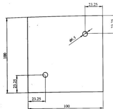
图 12.0.3 钢筋定位板示意图 (mm)
