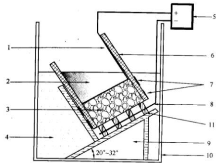
图 7.1.2 RCM 试验装置示意图
