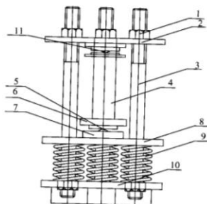
图 10.0.2 弹簧式压缩徐变仪示意图
