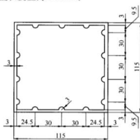
图 4.2.2 橡胶试件盒横截面示意图(mm)
