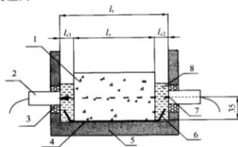
图 4.3.3-6 超声传播时间测量装置(mm)
