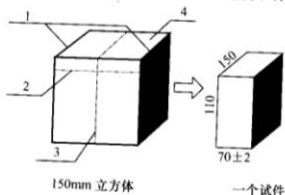
图 4.3.4 试件切割位置示意图(mm)
