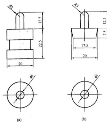
图 8.2.2-1 卧式收缩试验用测头 (mm)
