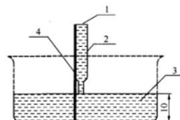
图 4.3.3-2 液面调整装置示意图 1—吸水管；2—毛细吸管；3—试验液体；4—定位控制装置
