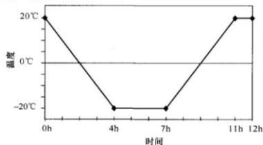
图 4.3.3-4 冻融循环制度
