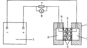
图 7.2.2-1 电通量试验装置示意图
