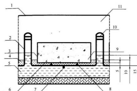
图 4.3.5 试件盒在单面冻融试验箱中的位置示意图 (mm)
