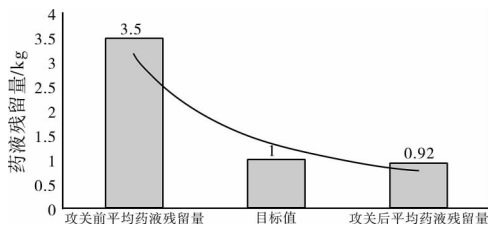
图 2 配料系统药液残留量攻关前后对比
